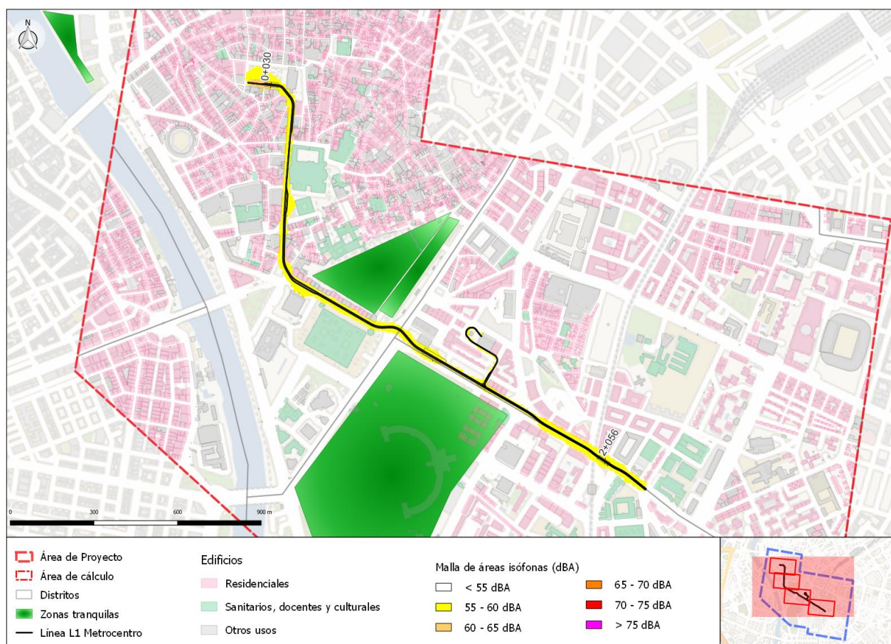
Ilustración 9. Mapa de curvas isófonas de la aportación sonora del METROCENTRO frente a las zonas tranquilas propuestas, Lden.
